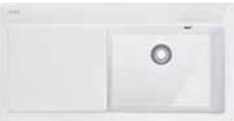
MTK 611-100 100 x 51 cm Väljalõige 98 x 49 cm (R=10 mm) Kauss 49,2/37,2/19 cm
