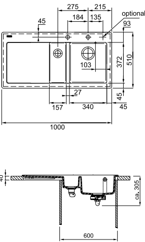
MTK 651-100 kauss paremal - Fraceram - Sõelkorv-ektsenterventiil 3½" - Vajutusnupp ümmargune rv - Sõelkorv-pruntventiil 1½" - 2 auku 35mm
