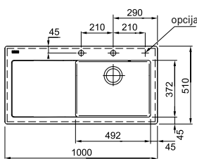
MTK 611-100 kauss paremal - Fraceram - Sõelkorv-eksenterventiil 3½"
