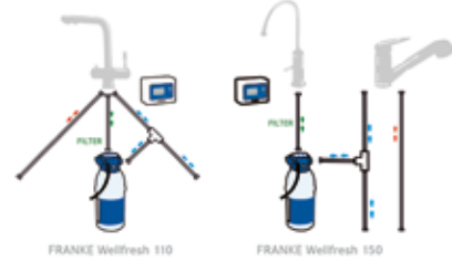
Ühendamise põhimõtteline skeem
