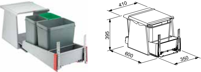
SORTER 700 CORNER 41 x 60 x 39,5 cm 4 5 6
